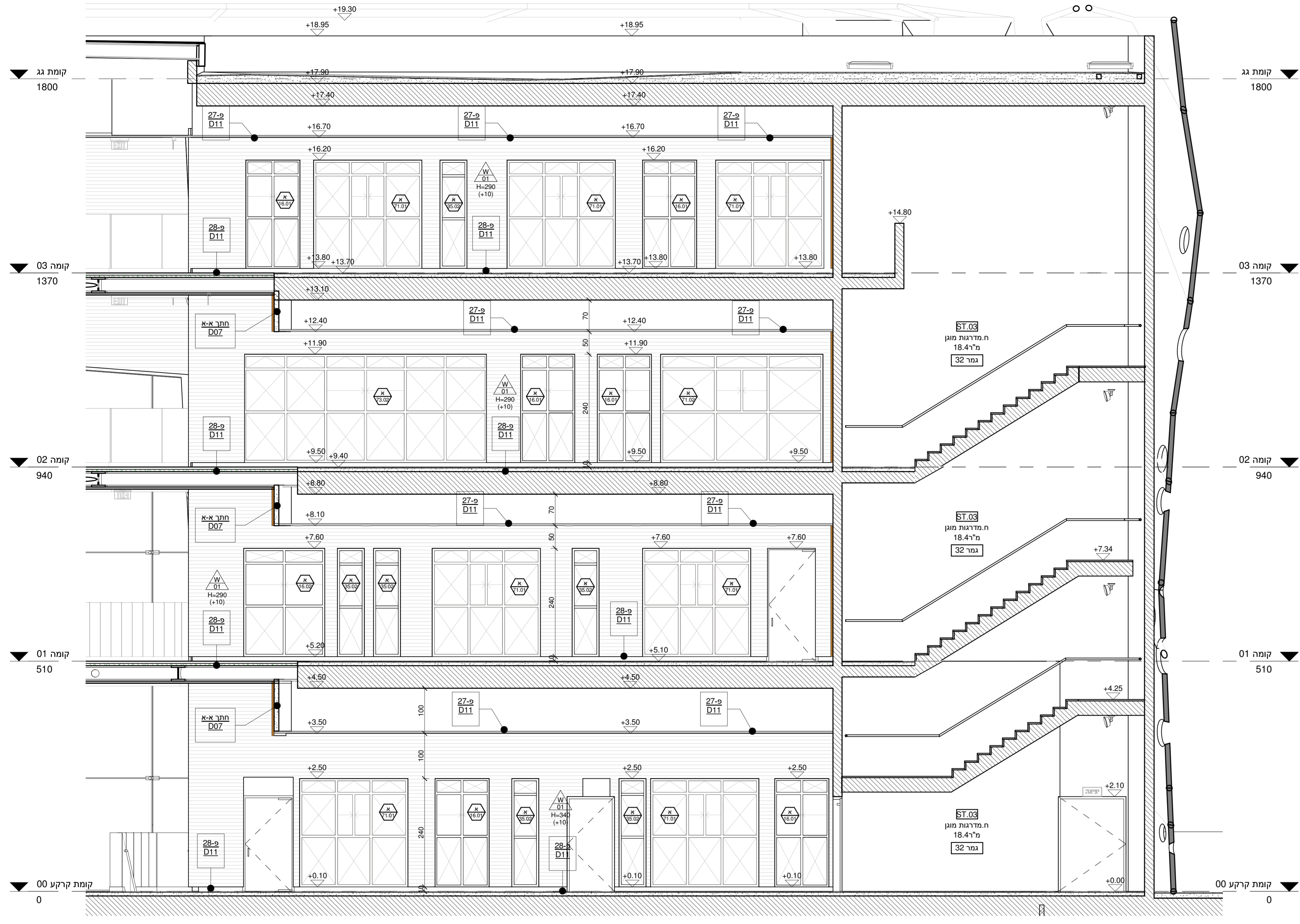
פריסת קיר מערבי מסדרון ב 1 : 50
