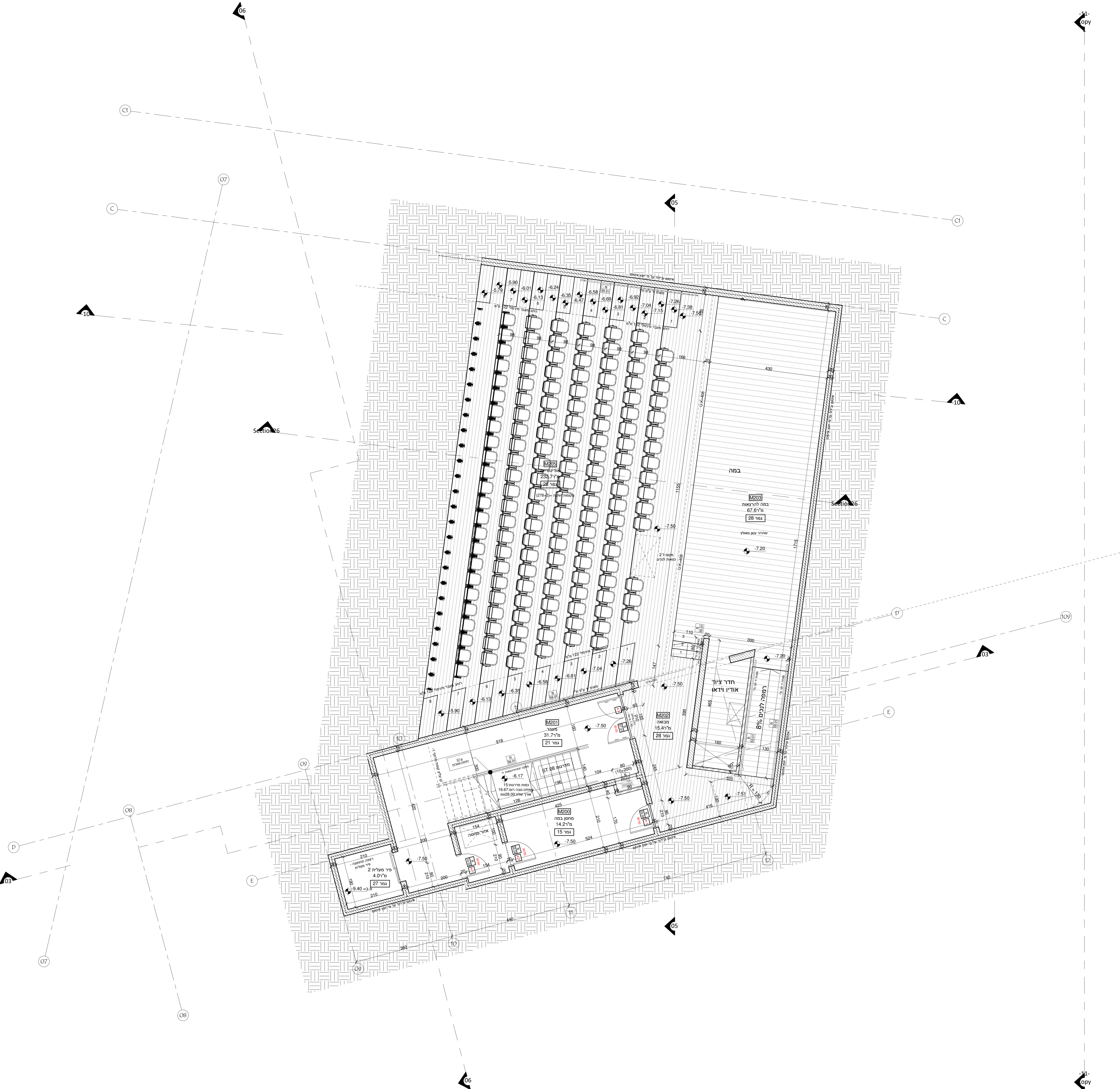
תוכנית קומת מרתף 2 - דרום 1 : 50
