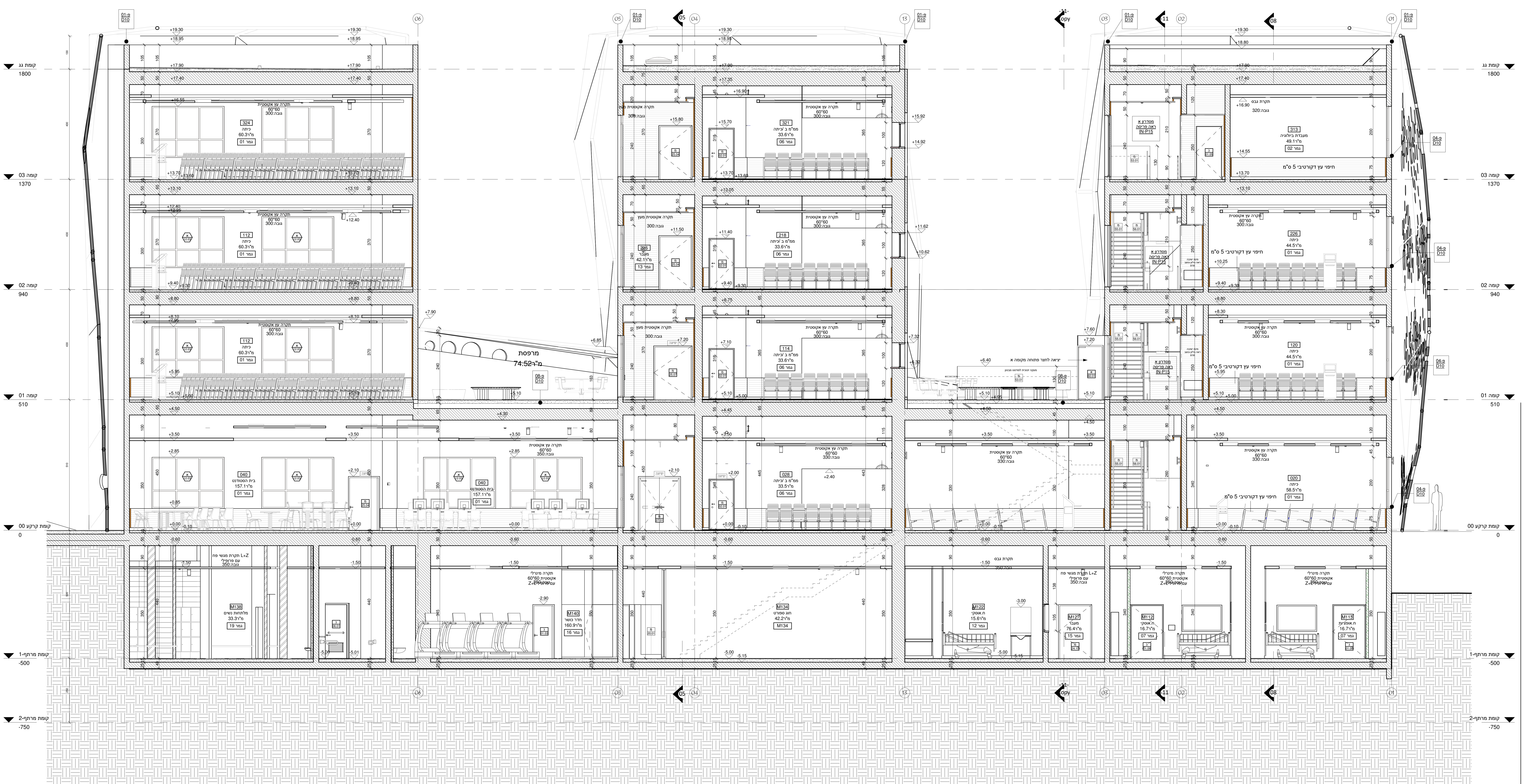
חתך 7-7 1:50
