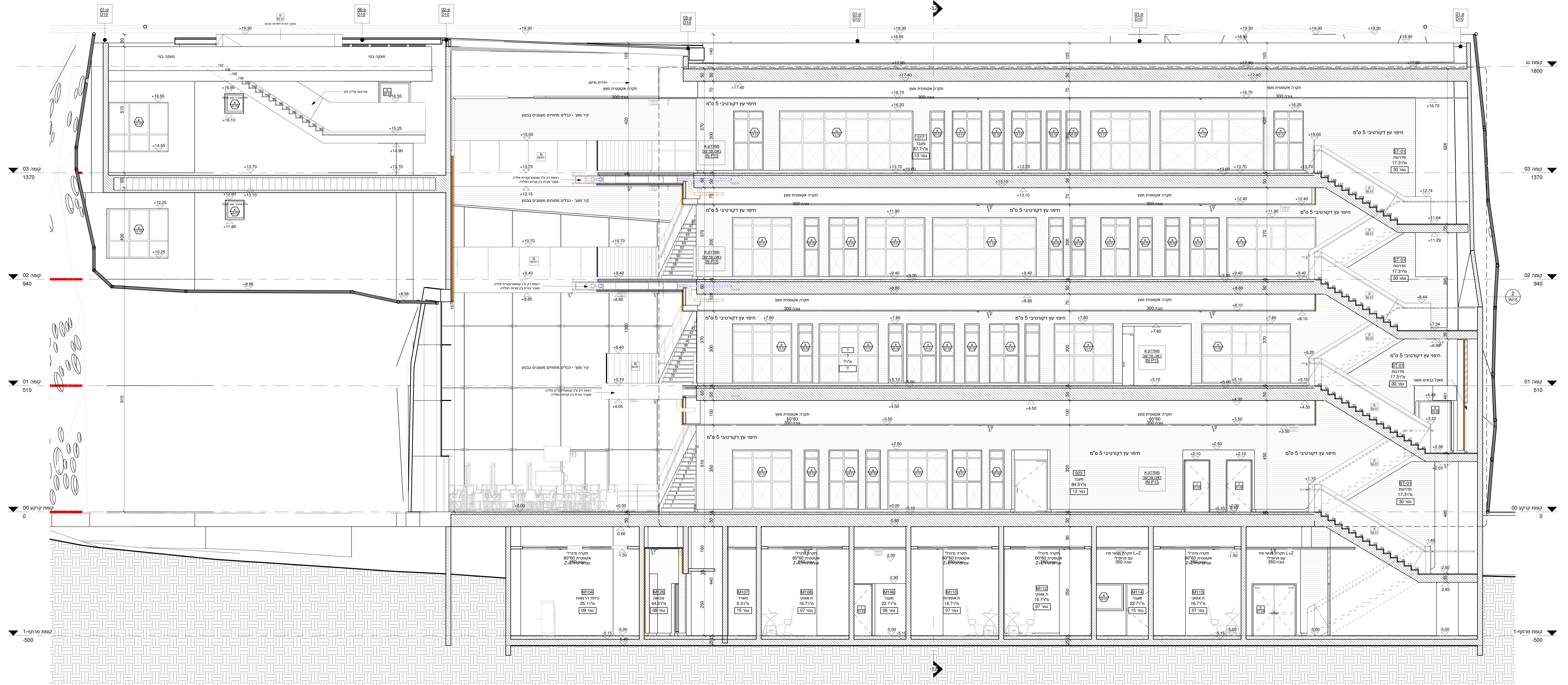
חתך 11-11 1 : 50
