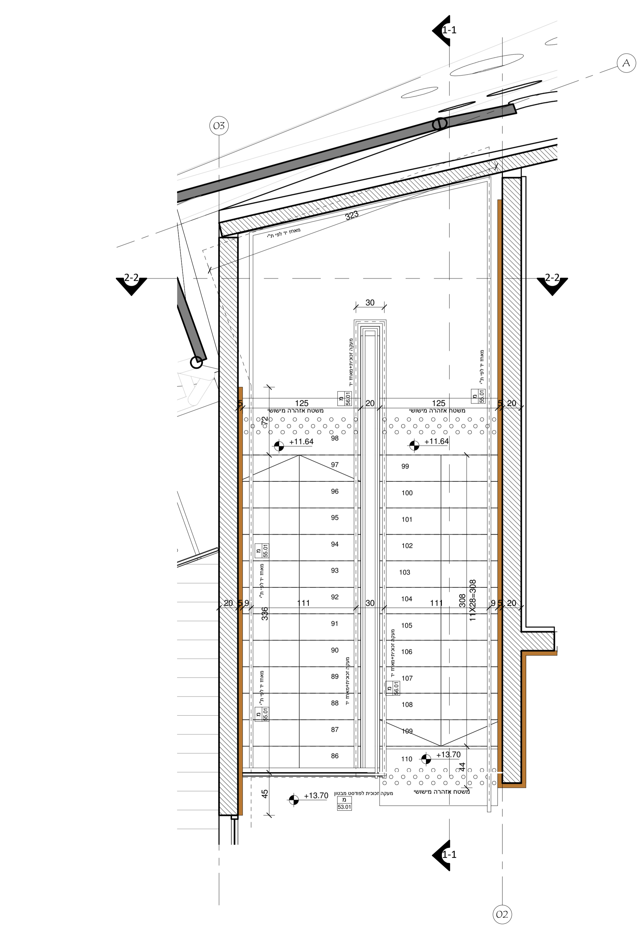
תוכנית מדרגות א_ מפלס +13.70 1 : 25
