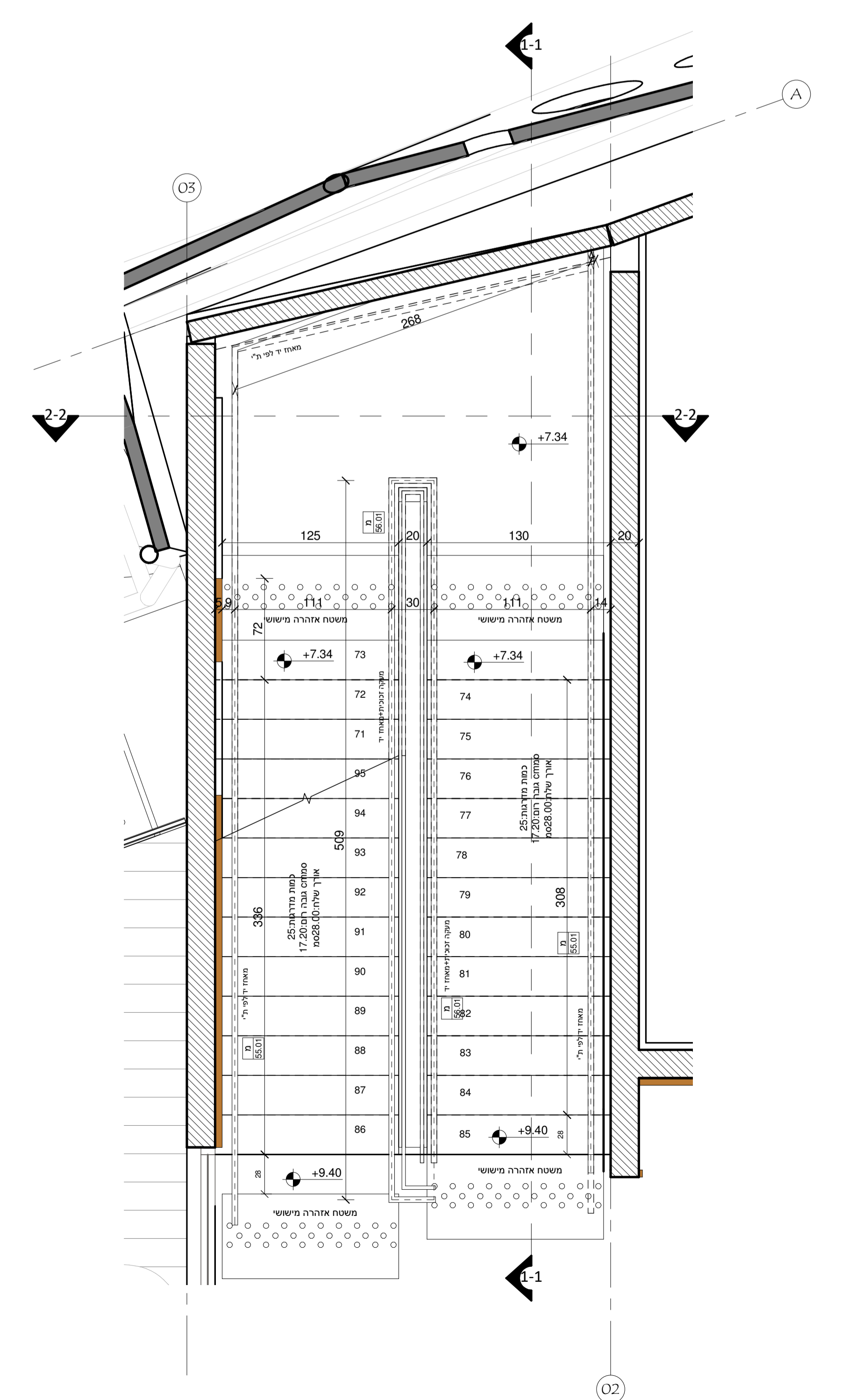
תוכנית מדרגות א_ מפלס +9.40 1 : 25
