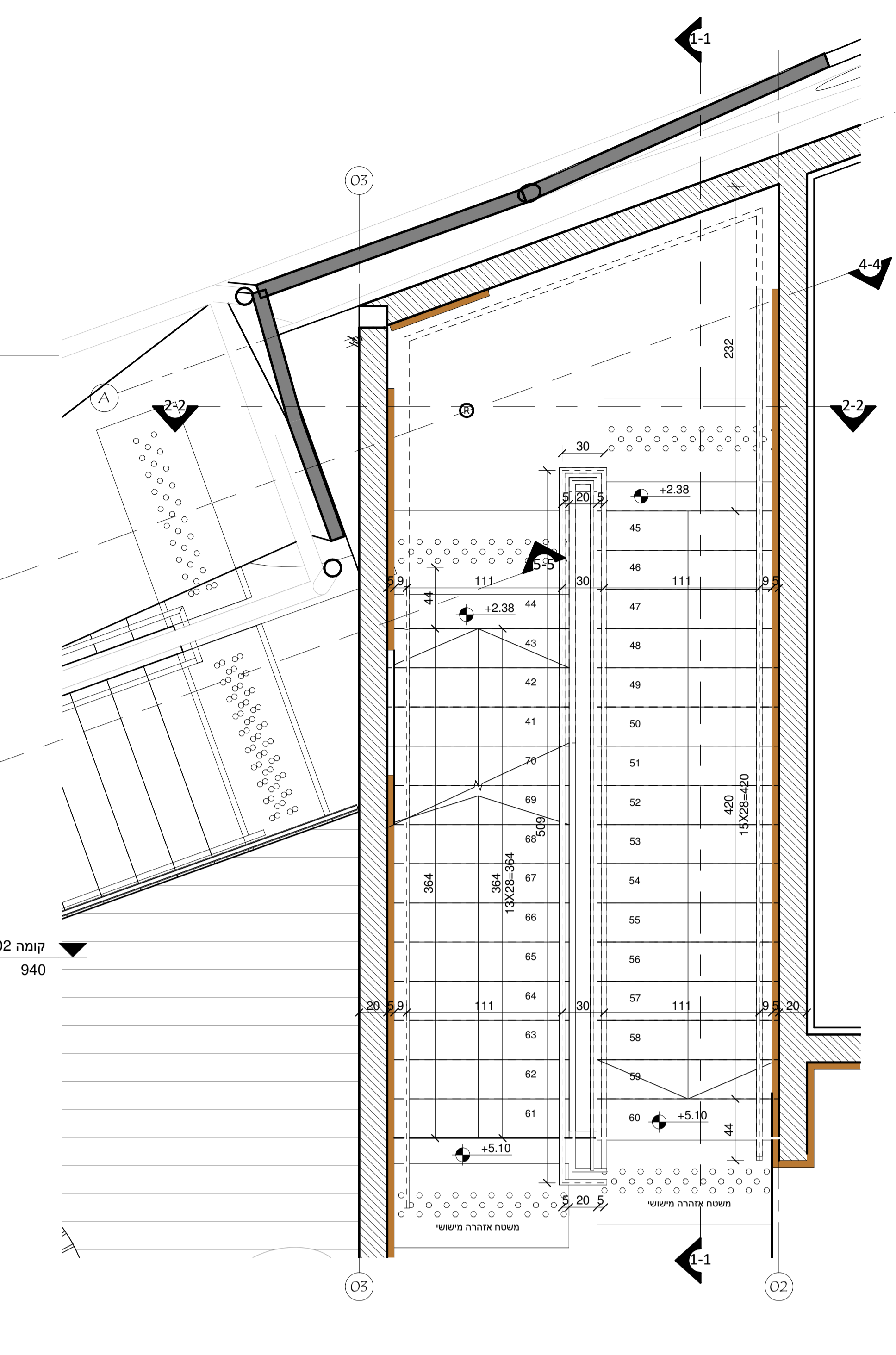
תוכנית מדרגות א_ מפלס +5.10 1 : 25
