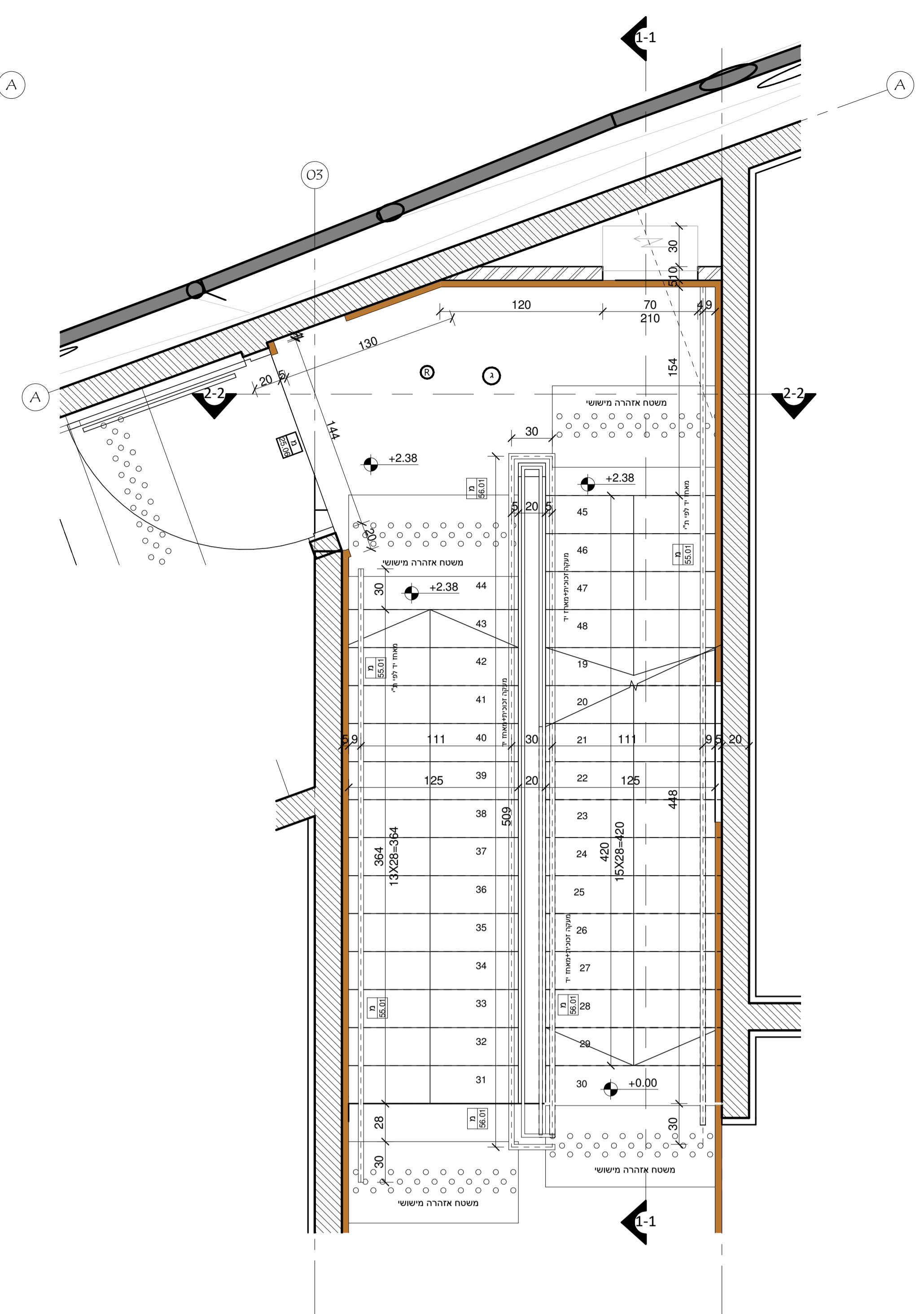
תוכנית מדרגות א_ מפלס 00 1 : 25
