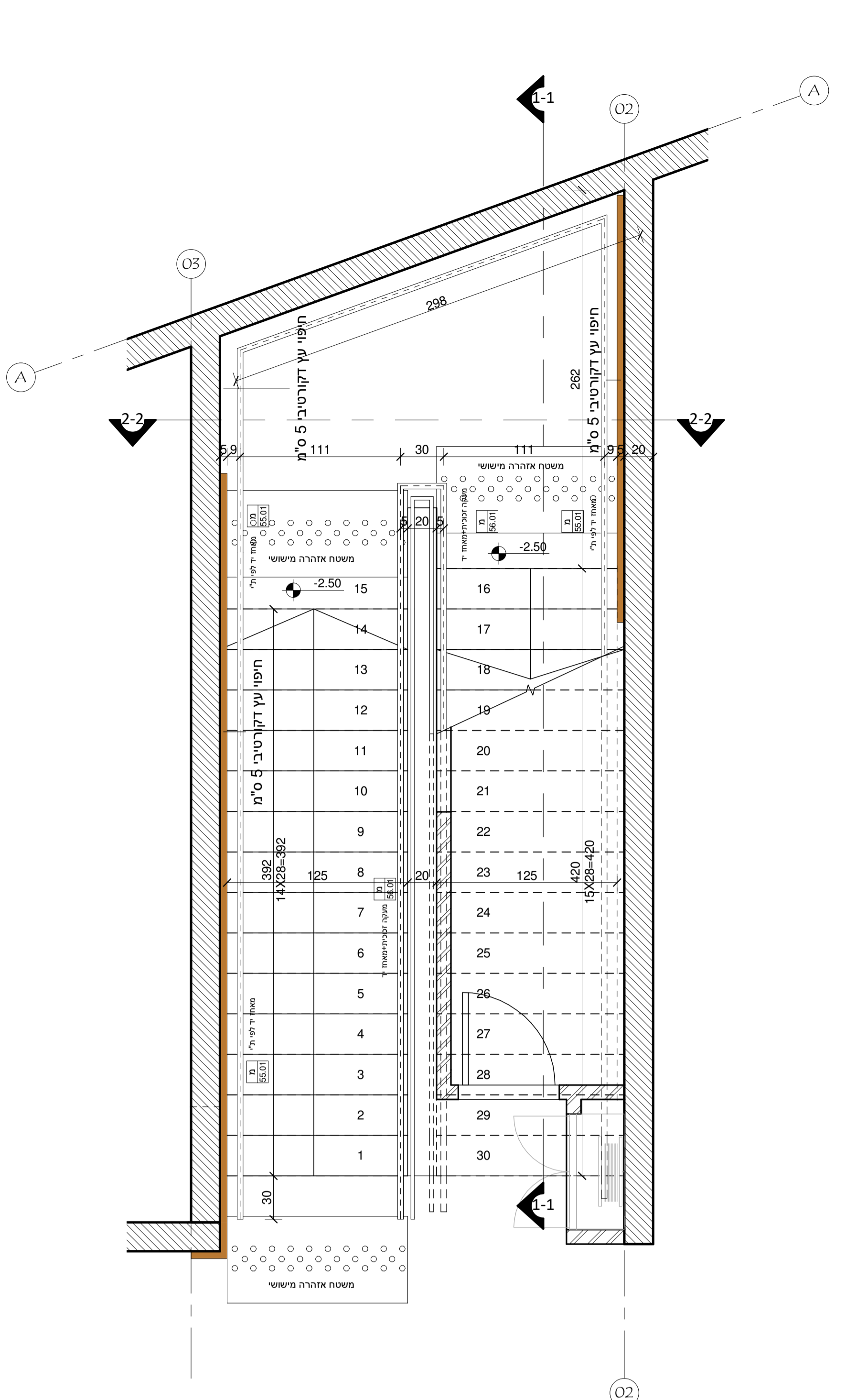
תוכנית מדרגות א_ מפלס -01 1 : 25
