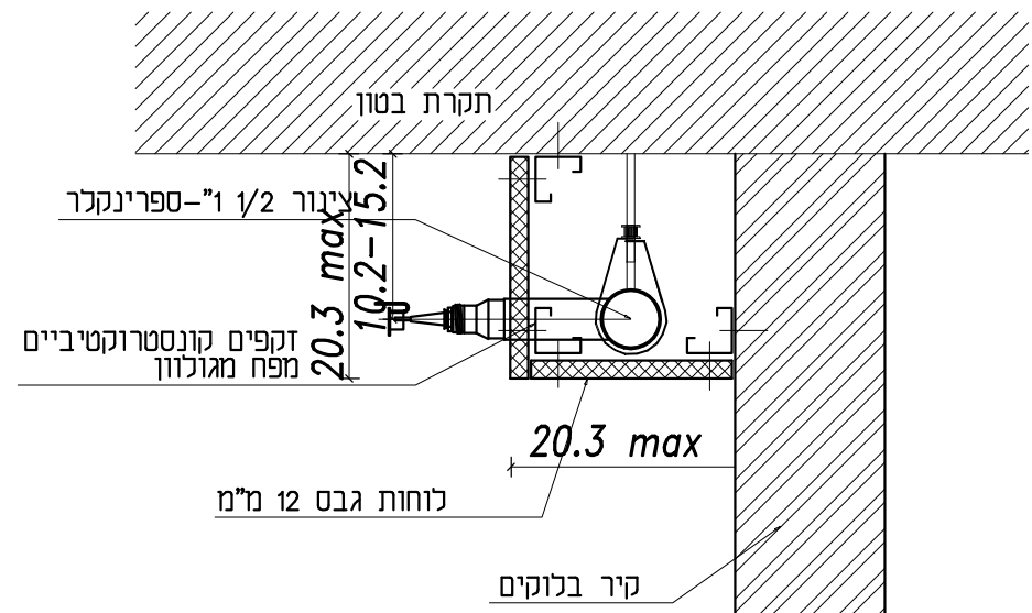
פרט SP1 פרט הנמכה לצינור ספרינקלר
