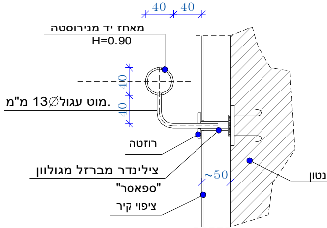
פרט מאחז יד - מדרגות
