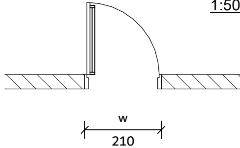
תוכנית 1:50
