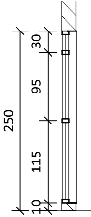
חתך 1:50
