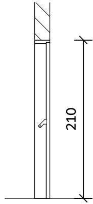
חתך 1:50
