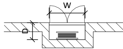
חזית 1:50
