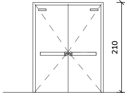
חזית 1:50
