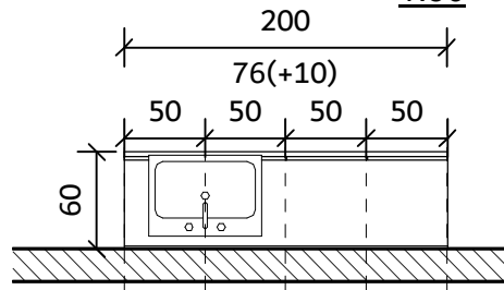
חזית 1:50
