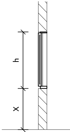
חתך 1:50
