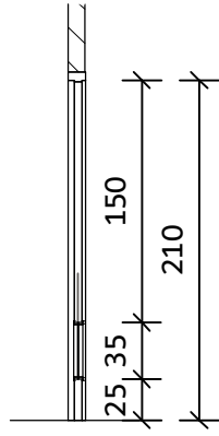
חתך 1:50
