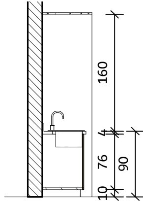
חתך 1:50
